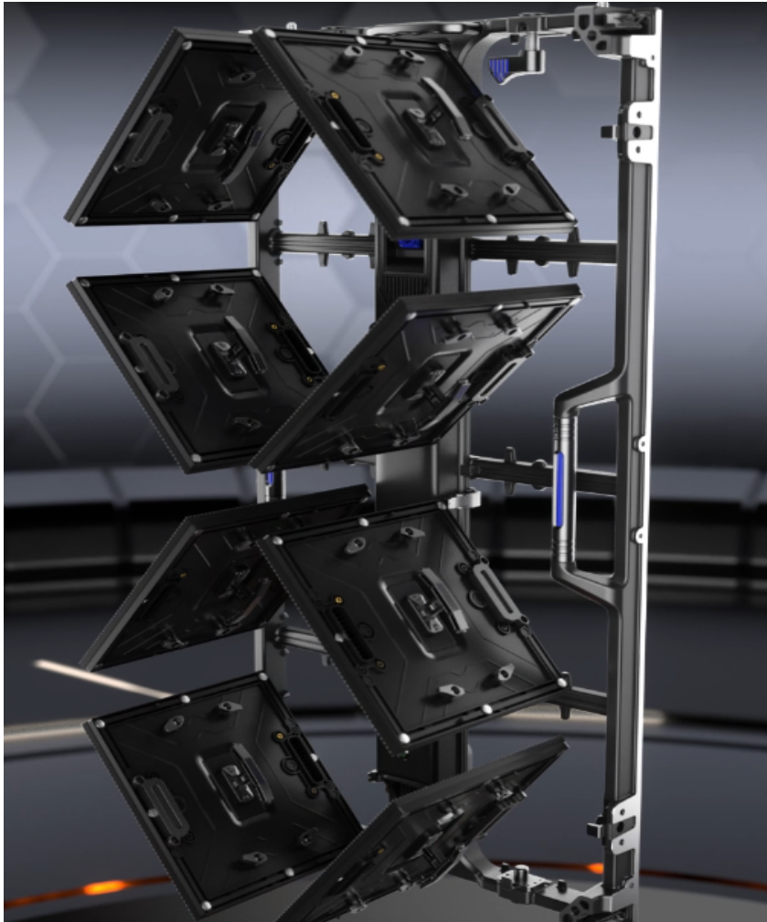
Easy module maintenance
